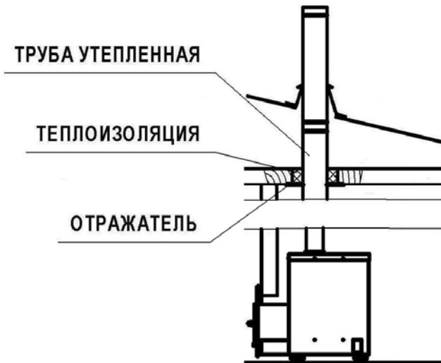
Рисунок 4. Монтаж дымохода сквозь потолок
